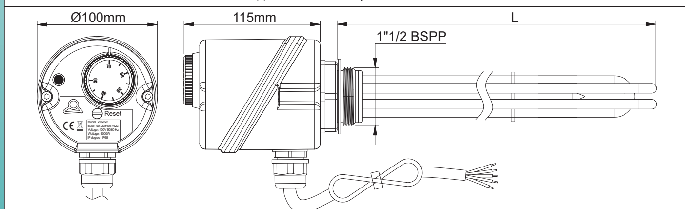
3-полюсный нагреватель 400 В
